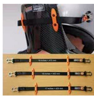
(A) trous de montage pour harnois mounting holes for harness
